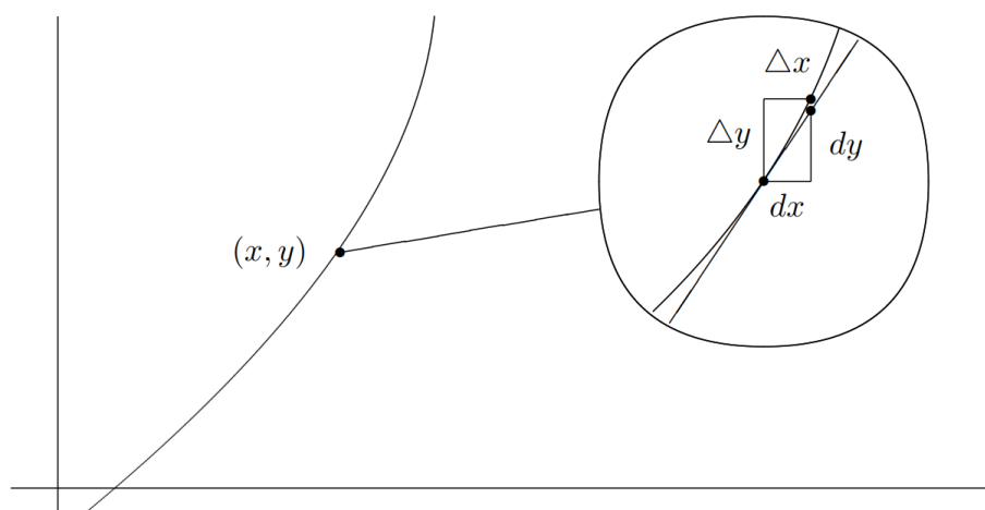
Figura 2 Microscopio infinitesimo con fattore di scala \frac{1}{dx} centrato in (x, y) (tratta da Keisler, 1976b, p. 37).
