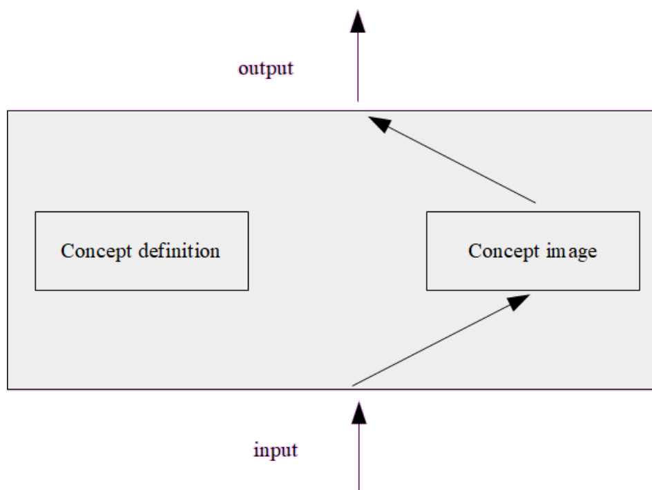
Figura 4 Mancata interazione tra concept-image e concept-definition nel caso di risposta intuitiva (tratta da Vinner, 1991, p. 73).
