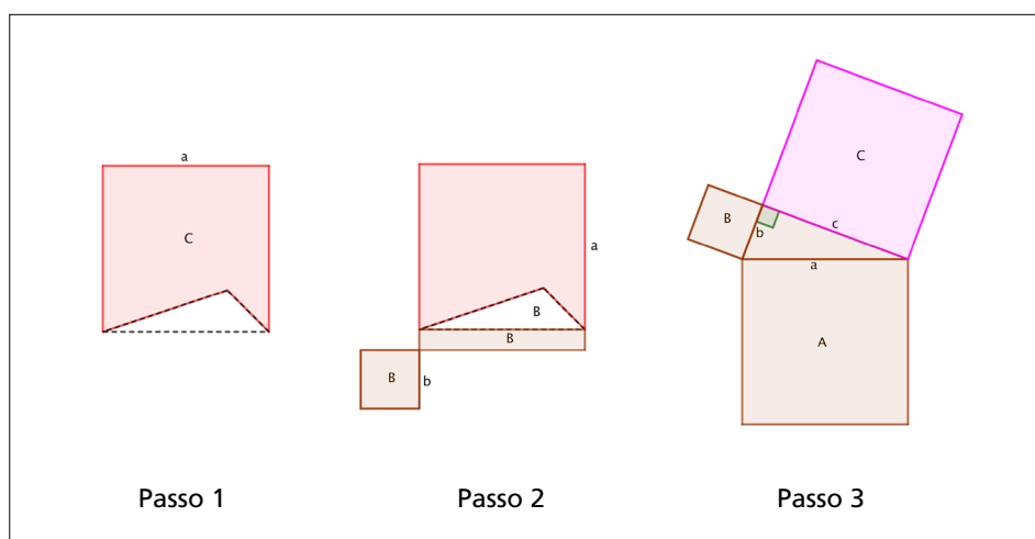
Figura 10 Quadratura del pentagono di area C .
