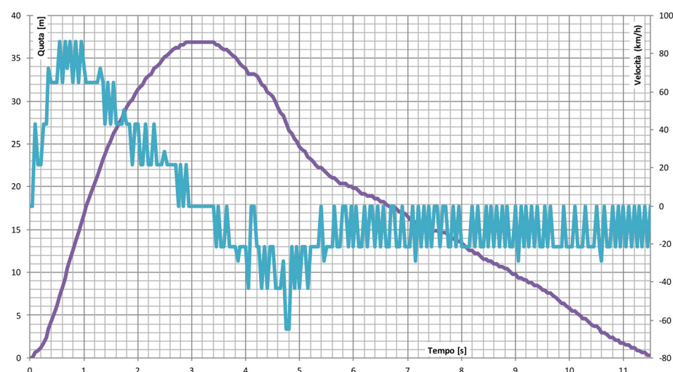
Figura 18 Grafico quota e velocità di un razzo-modello generato con foglio di calcolo dai dati acquisiti con l'altimetro: altitudine (viola) e velocità (azzurro) nel tempo.
