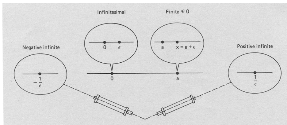
Figura 1 Microscopi infinitesimi con fattore di scala \frac{1}{\epsilon} centrato in 0 e in un numero reale a e telescopi infiniti puntati su \frac{1}{\epsilon} e -\frac{1}{\epsilon} (tratta da Harnik, 1986, p. 45).
