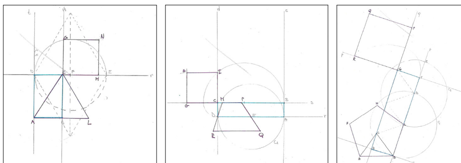
Figura 18 Quadratura del triangolo isoscele, del trapezio e del pentagono regolare.
