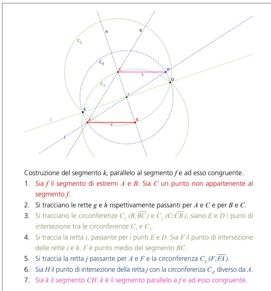
Figura 1 Costruzione con riga non graduata e compasso "collassante" o "molle".
