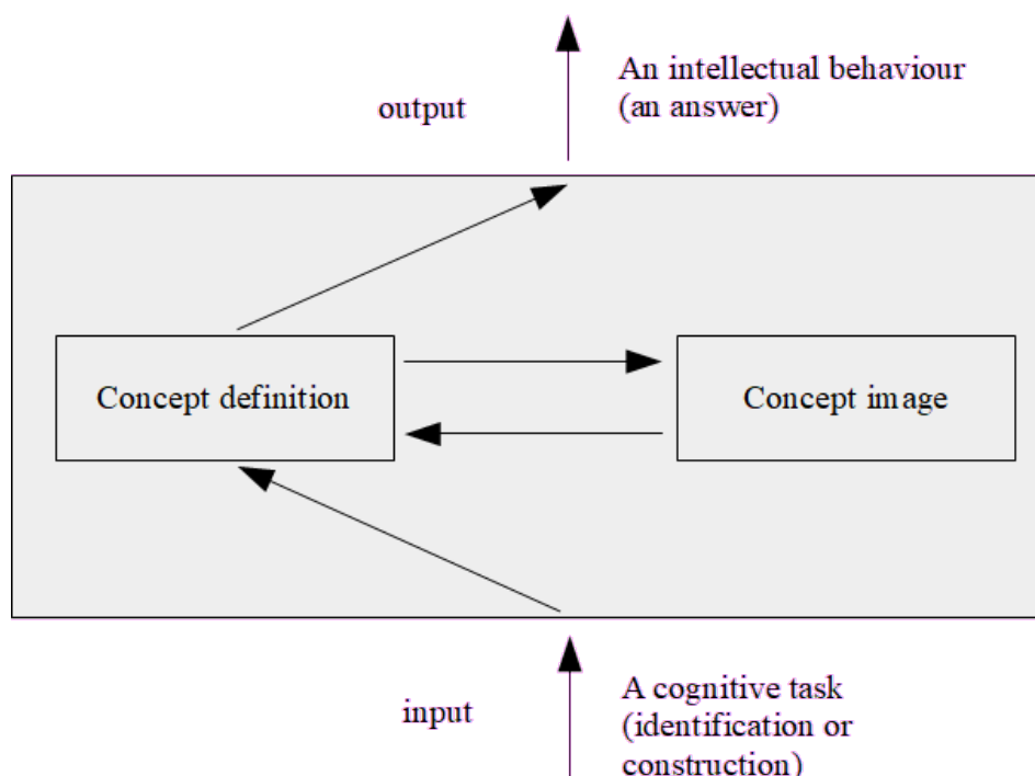
Figura 3 Interazione ideale tra concept-image e concept-definition (tratta da Vinner, 1991, p. 71).
