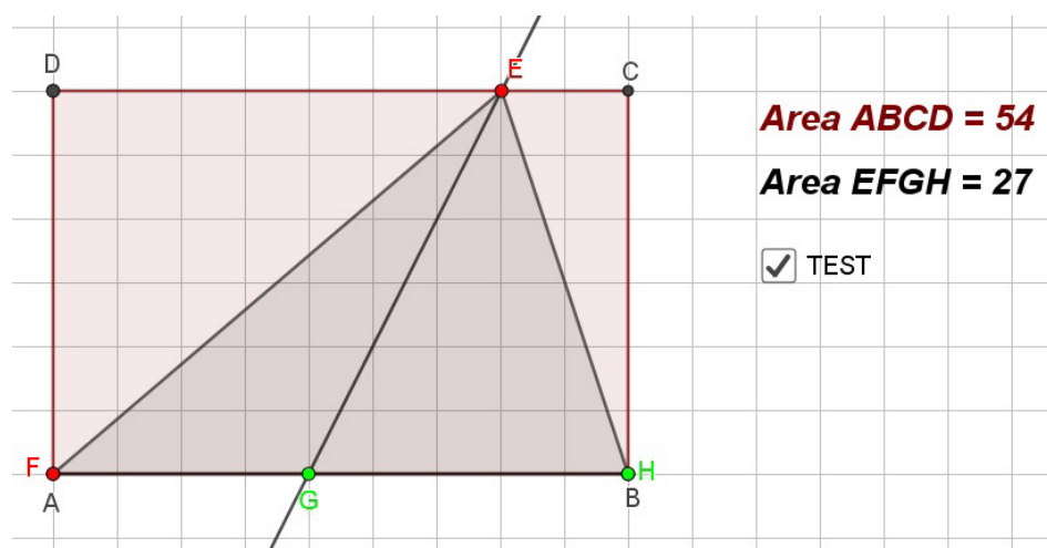
Figura 11 Esplorazione di un caso degenere.
