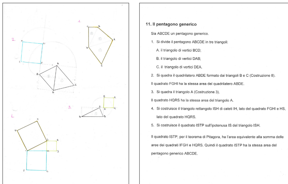
Figura 20 Quadratura del pentagono generico e passi della costruzione.
